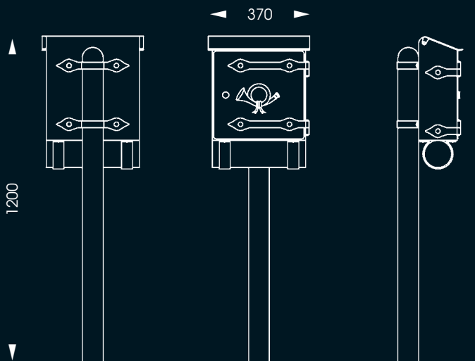
B 8484 BRIEFKASTEN MIT ZEITUNGSROLLE FREE STANDING BOX FOR MAIL AND NEWSPAPER
