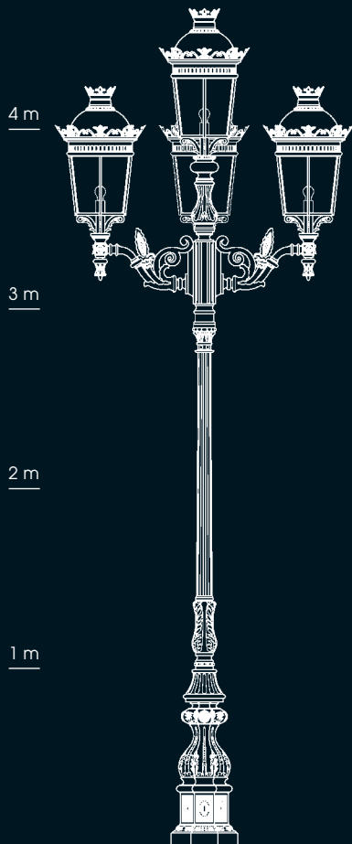
POLE M 316 BRACKET KR 440 LAMP AL 1535-N
